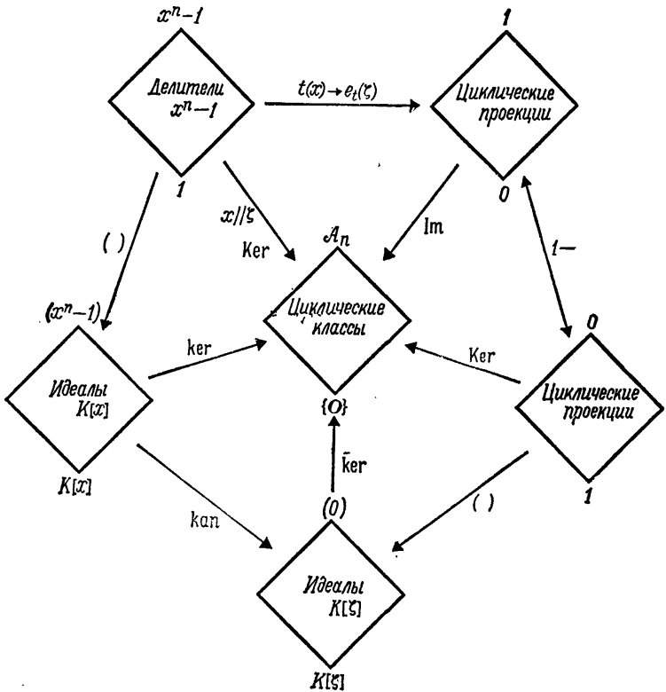
Рис. 61. Основная диаграмма. [x//\zeta] обозначает подстановку x \rightarrow \zeta .
